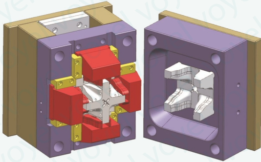
Plastik Enjeksiyon Kalıbı
