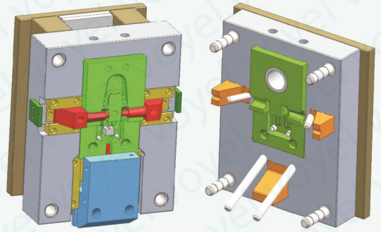
Metal Enjeksiyon Kalıbı
