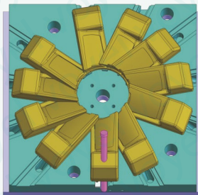
Plastik Pervane Kalıbı
